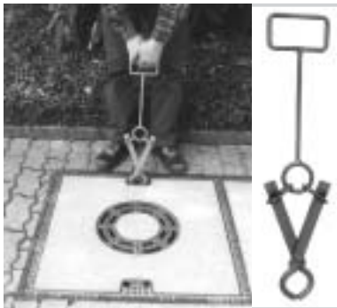
Hand-Zange für Kabelschächte
